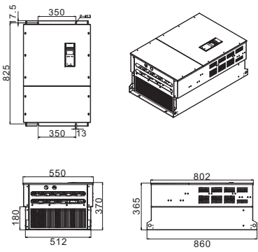
框号8 : YD3185 T4(B)N YD3200 T4(B)N YD3220 T4(B)N YD3250 T4(B)N
