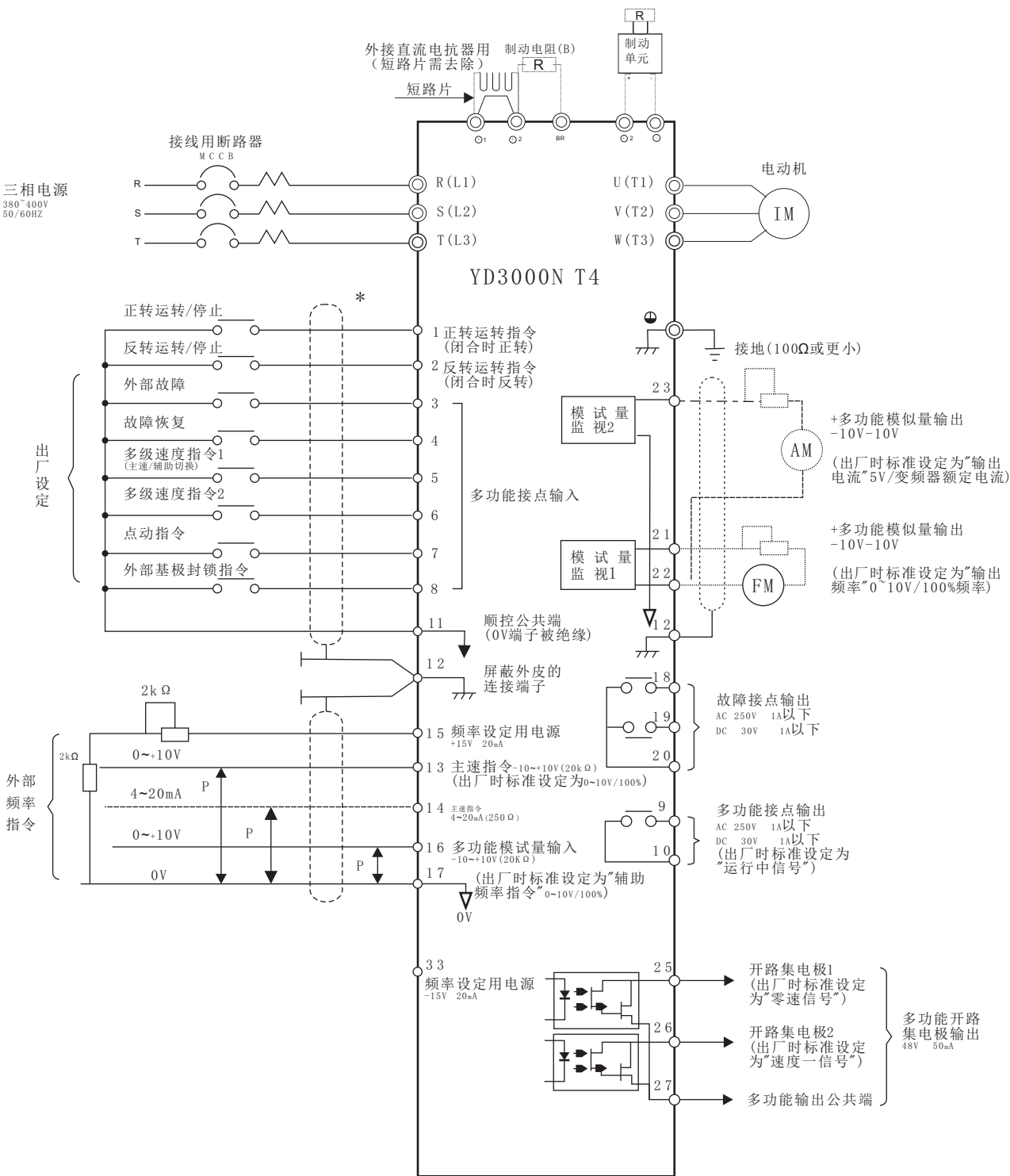
连接图(以YD3185 T4 BN 为例)
